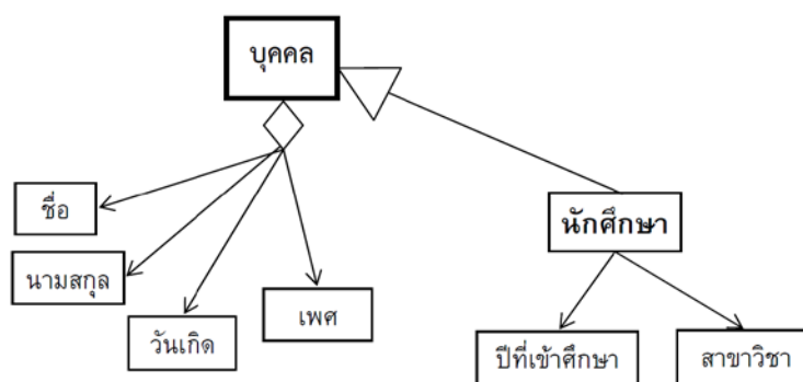
รูปที่ ๑ ตัวอย่างแบบจำลองข้อมูลบุคคล (Data Model) ในรูปแบบของ UML Class Diagram
